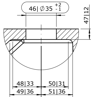
Pormenor C Escala 2 : 5
