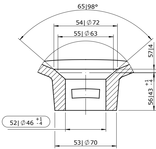
Pormenor D Escala 2 : 5
