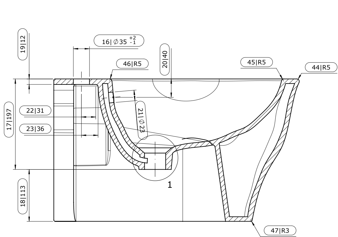
Corte A-A
