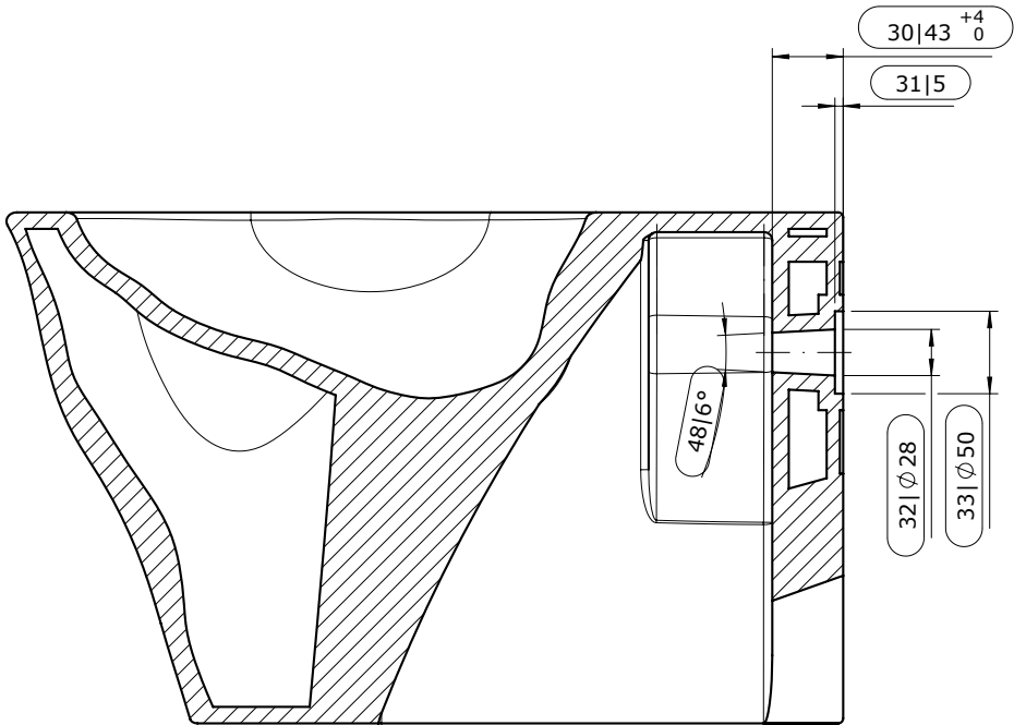
Corte C-C
