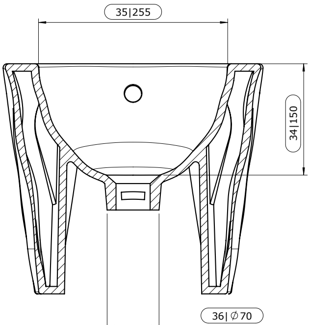
Corte B-B
