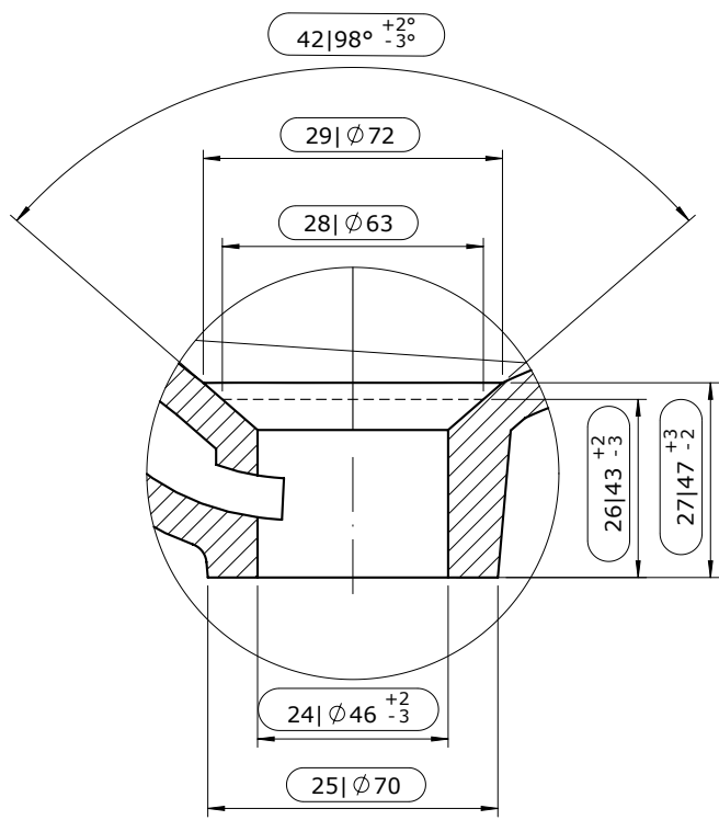
Pormenor 1 Escala 1 : 2
