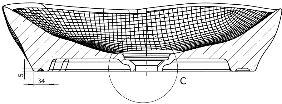
Corte B-B
