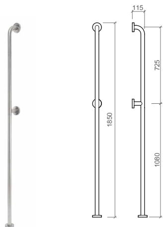
42967 Barre d'appui
