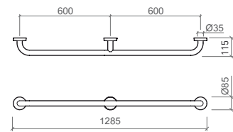
42966 Barre d'appui 120
