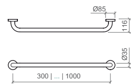
42972 Barre d'appui 100
